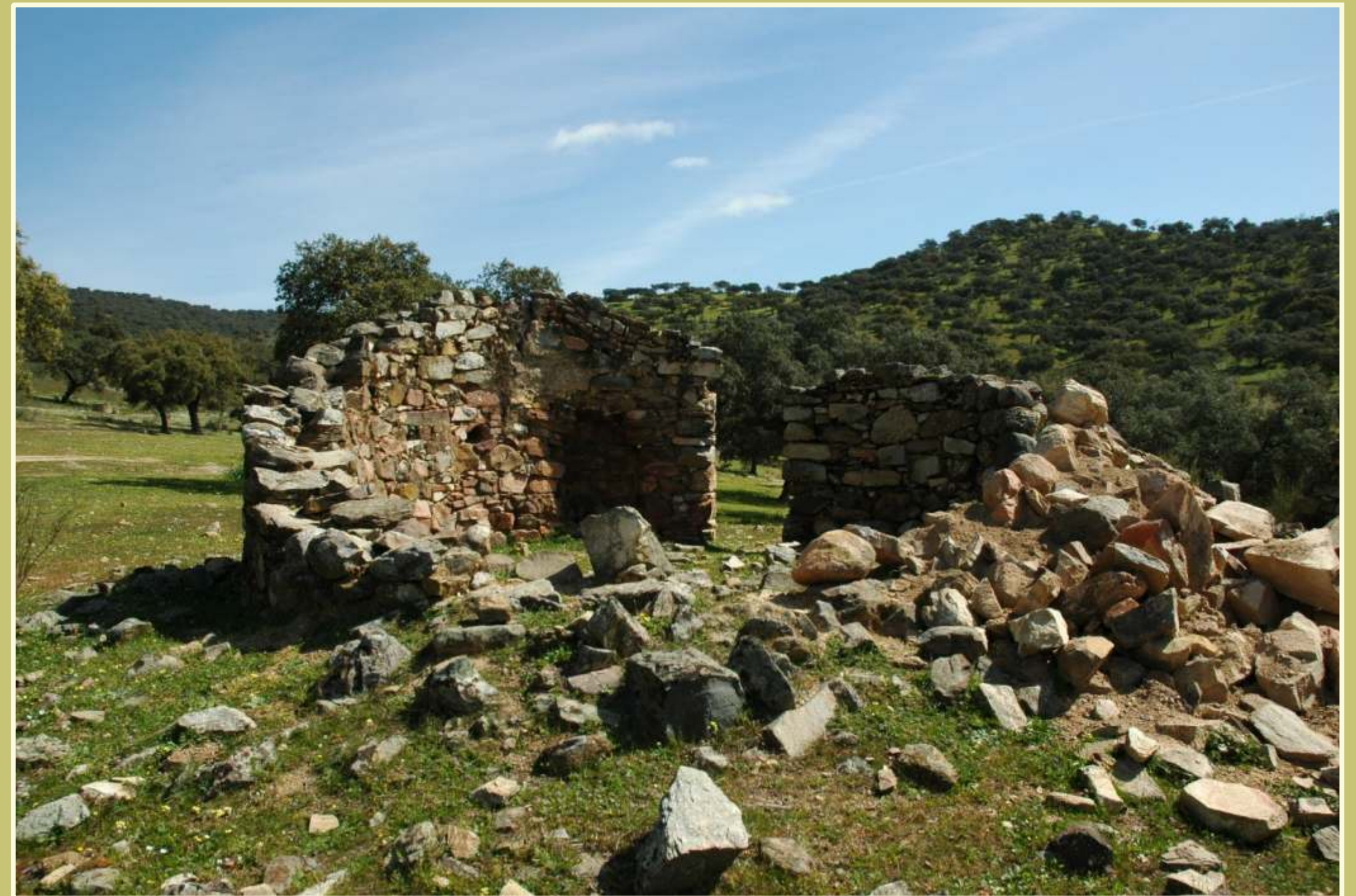
Restos de vivienda en Sierra Morena. Puede observarse la técnica constructiva de mampostería con rocas autóctonas (cuarcitas, granito y pizarras).
